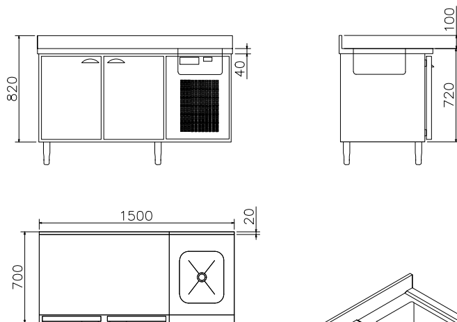
REFRIGERADOR / FREEZER HORIZONTAL 02 PORTAS CORPO EXTERNO E PORTAS EM AÇO INOX 304 CORPO INTERNO EM ALUMÍNIO POTÊNCIA: 0,45kw - 160W/0F. PÉS COM SAPATA DE ALTURA AJUSTÁVEL
